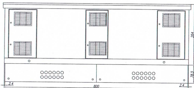
ELEWACJA FRONTOWA
