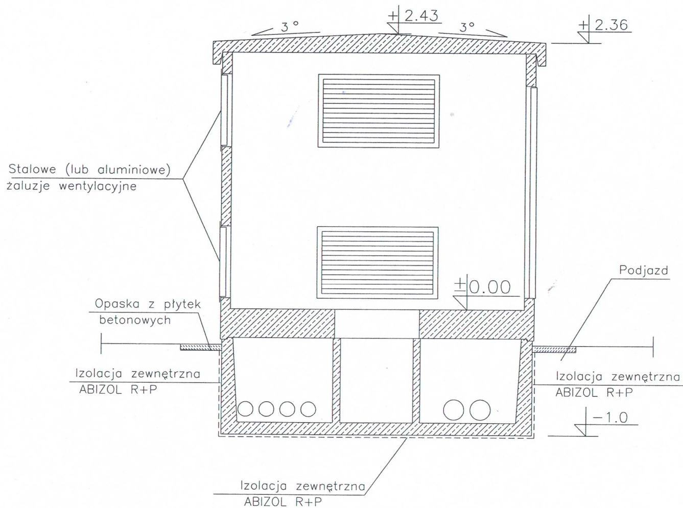
RZUT 5-5 PRZEKRÓJ POPRZECZNY 1:30
