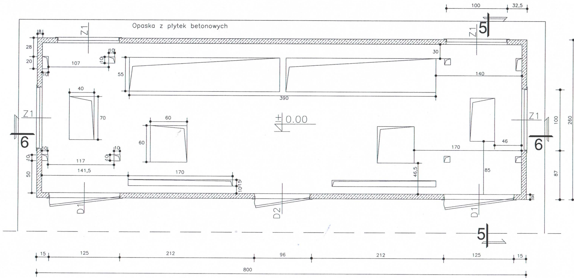
RZUT PRZYZIEMIA 1:35
