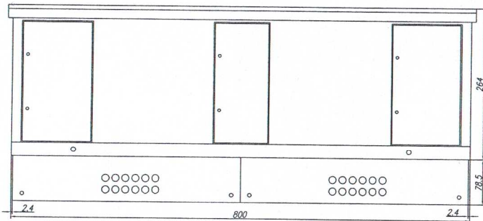
ELEWACJA FRONTOWA
