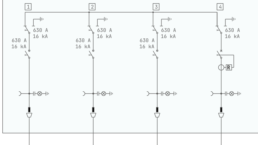
Rozdzielnica SN typu Xiria / Xiria-xGear w układzie KKKT; 630A, 24kV, 16kA, IP3X
