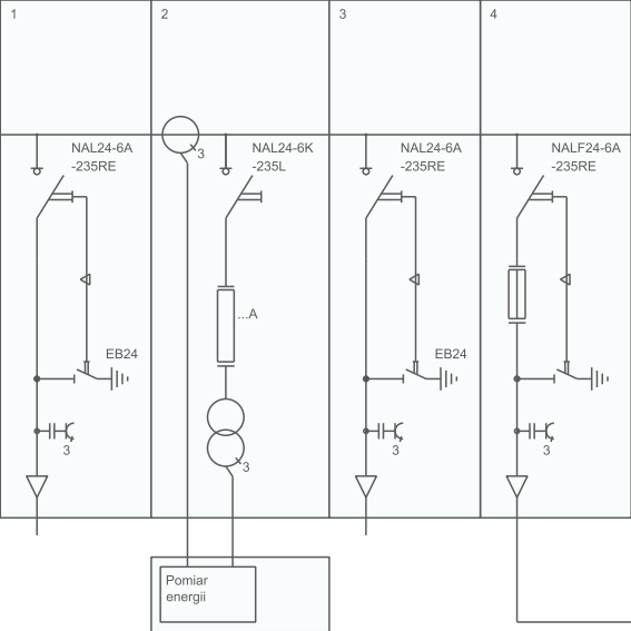
Rozdzielnica SN typu RSL 630A; 24kV; 20/50kA, IP4X
