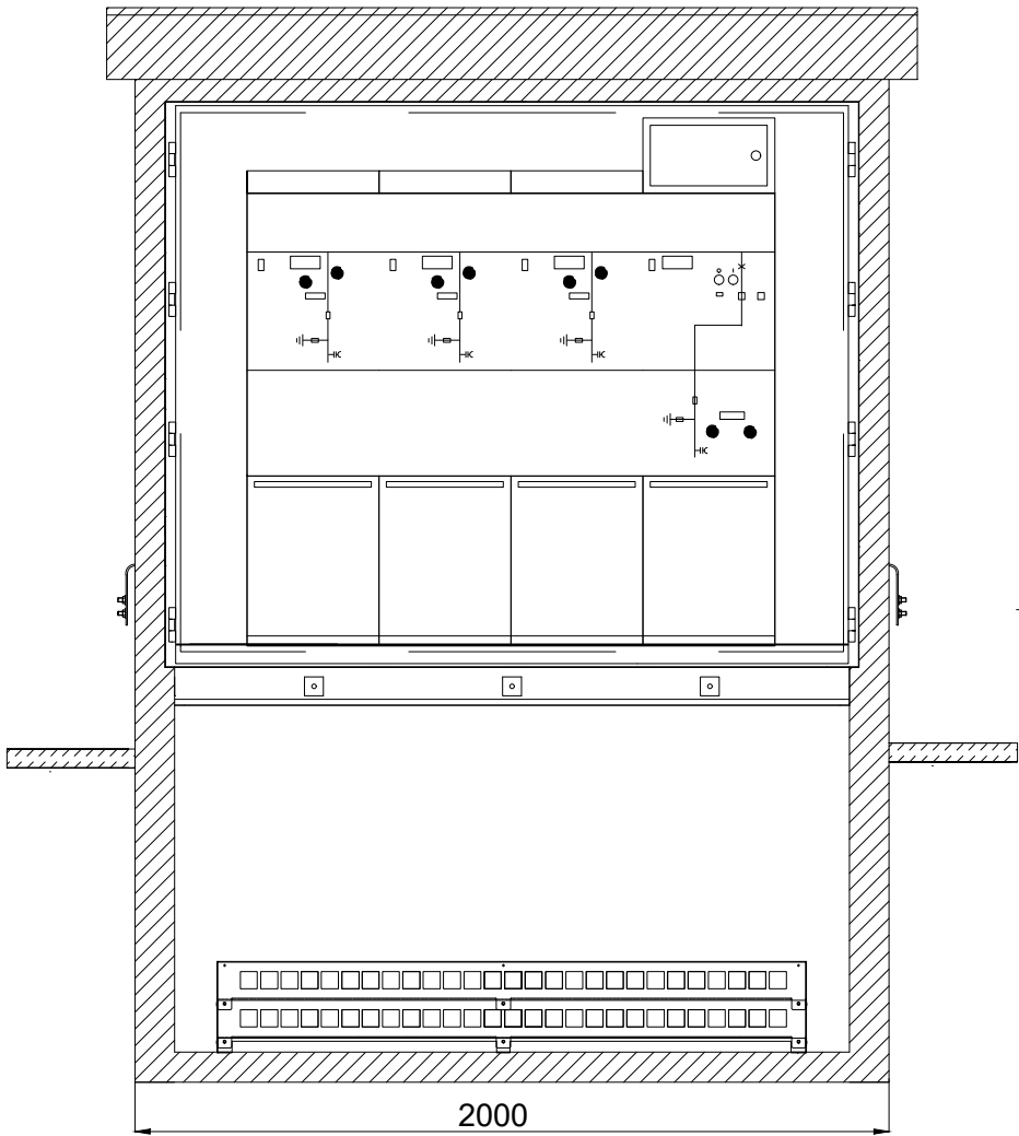
PRZEKRÓJ A - A
