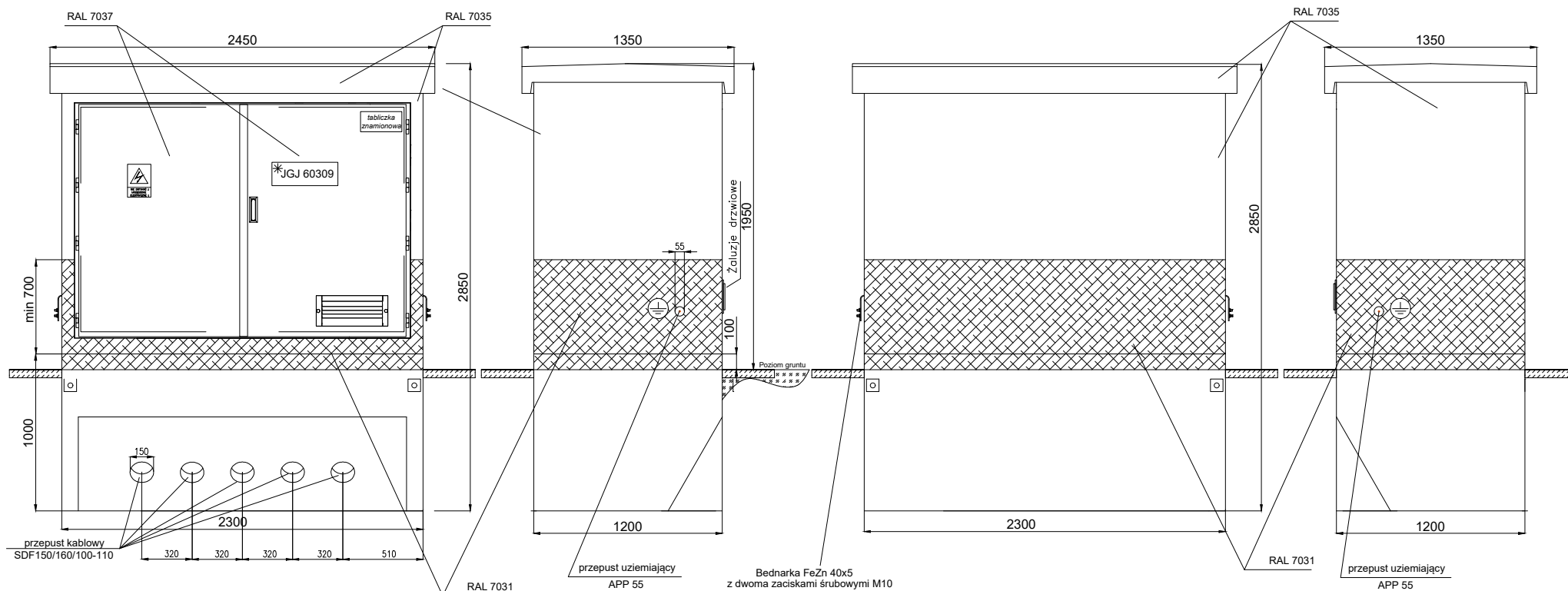
ELEWACJA FRONTOWA
